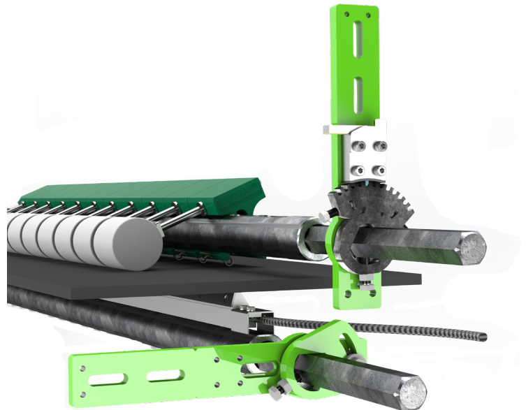
Fördergurtabstreifer Serie 520
