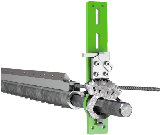
Fördergurtabstreifer Serie 830
