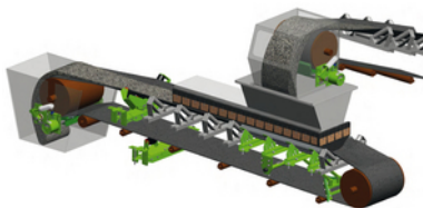
Komplette Bandanlage mit Elementen aus der Reihe des STARCLEAN® Baukastensystems
